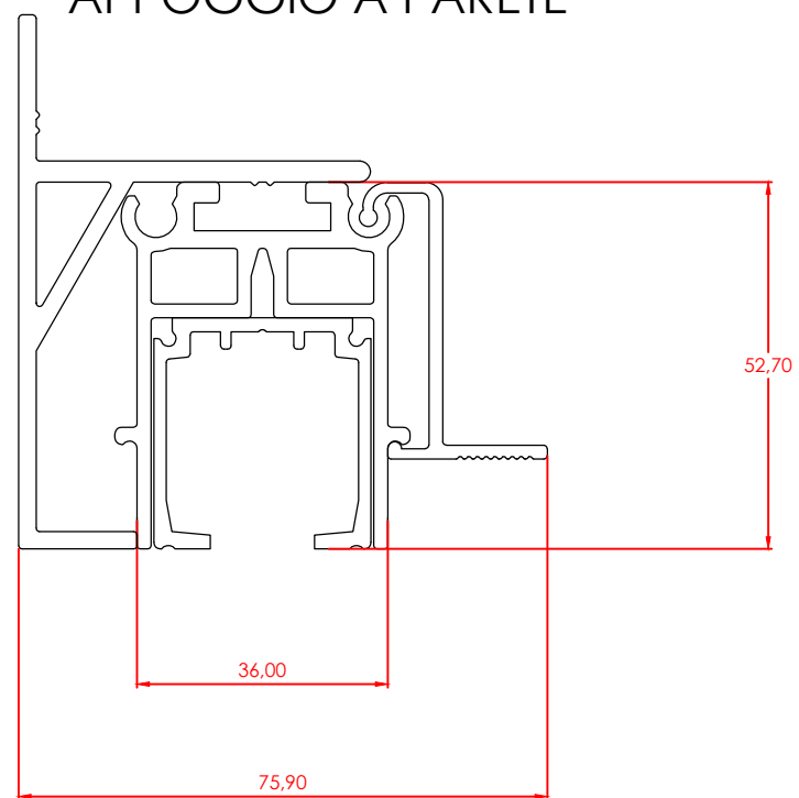
BINARIO DA AFFOGARE A SOFFITTO, PROFILO CON APPOGGIO A PARETE
