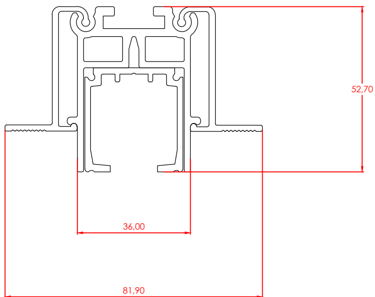
BINARIO DA AFFOGARE A SOFFITTO, PROFILO SENZA APPOGGIO A PARETE
